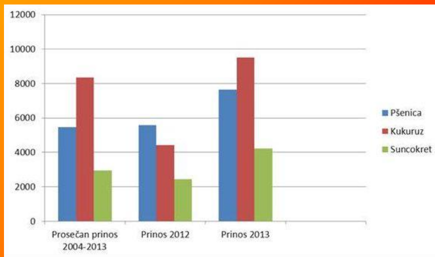
Grafikon 1: Prosečni prinos pšenice, kukuruza i suncokreta u Srbiji
